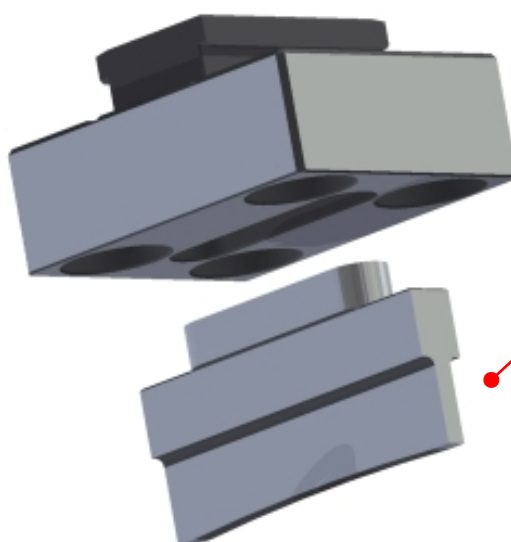
Punzón Punch
