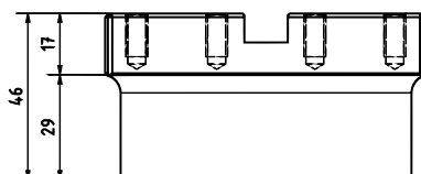
Cuchilla TC / TC Blade
