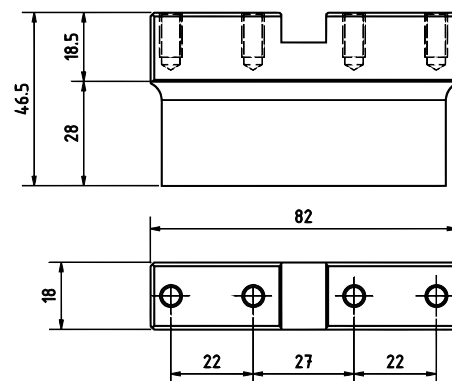
Cuchilla Estándar / Standard Blade
