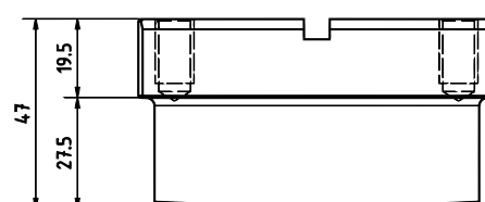
Cuchilla WT / WT Blade
