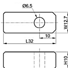
Estación E Superior mod.1 Station E Upper Key mod.1
