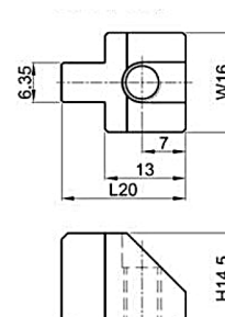
Estación D Inferior mod.2 Station D Lower Key mod.2
